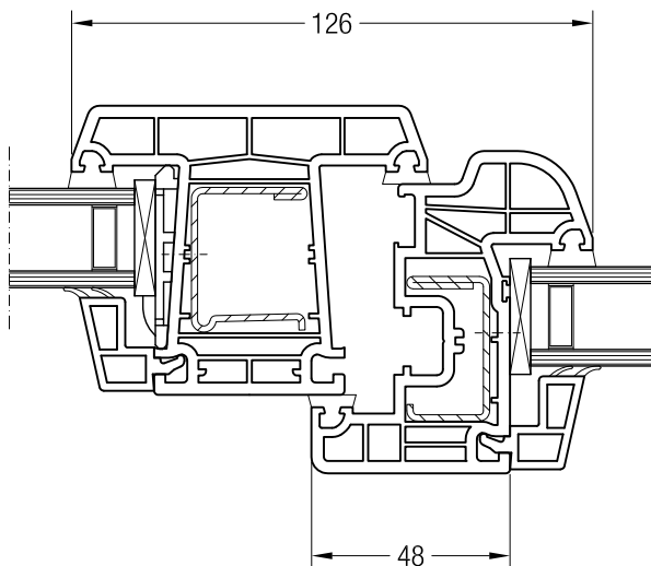
Импост 86, 1550020 и створка 48 круглая, 1550481
