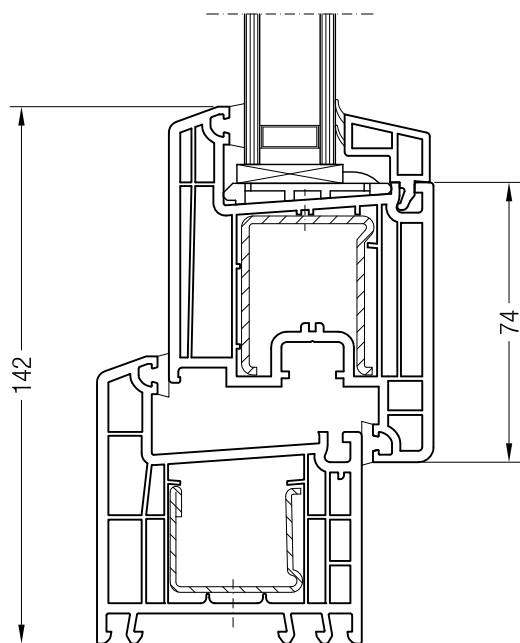
Коробка 76-2, 1550950 и створка Z 74, 1550510
